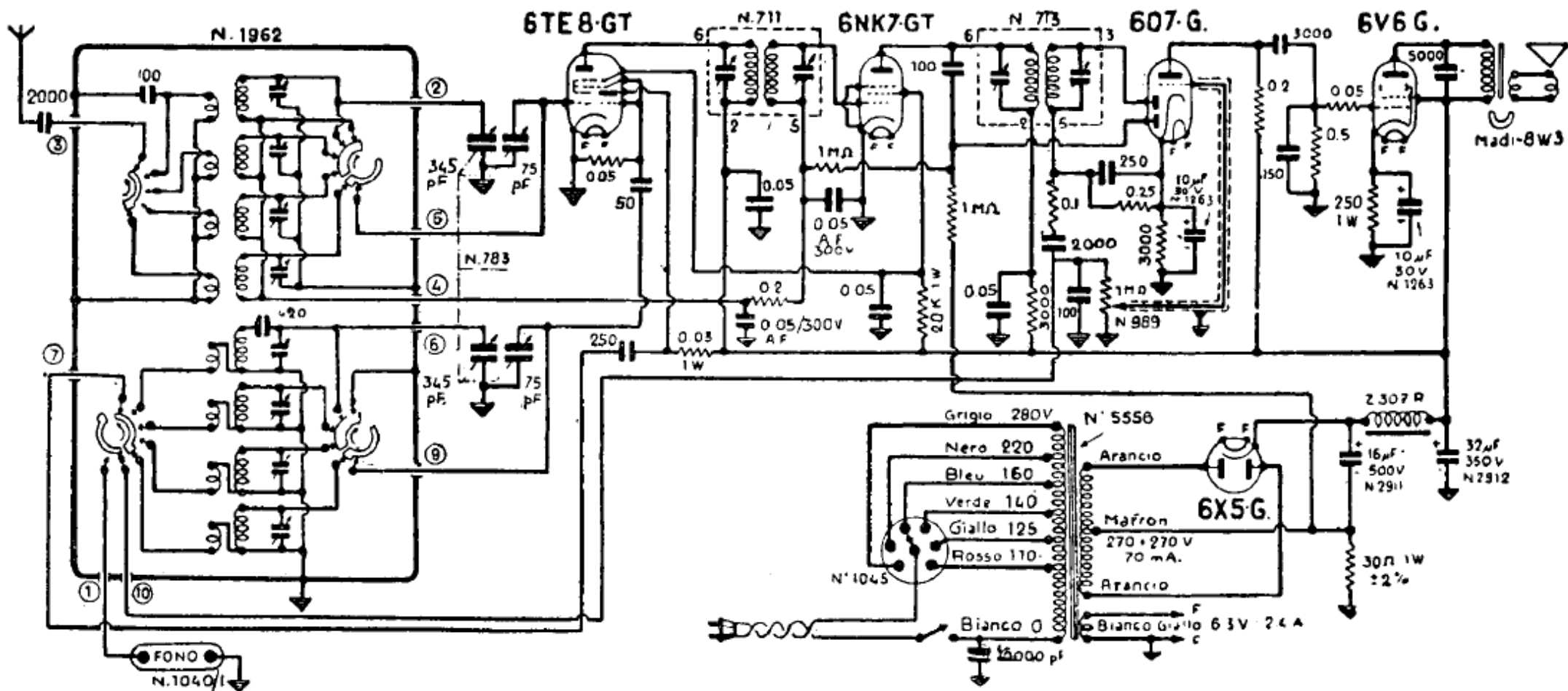
GELOSO. — Mod. G. 75 R. — 12,5-21 m; 21-34 m; 34-54 m; 190-580 m. — MF: 467. — Produzione 1946-47.
